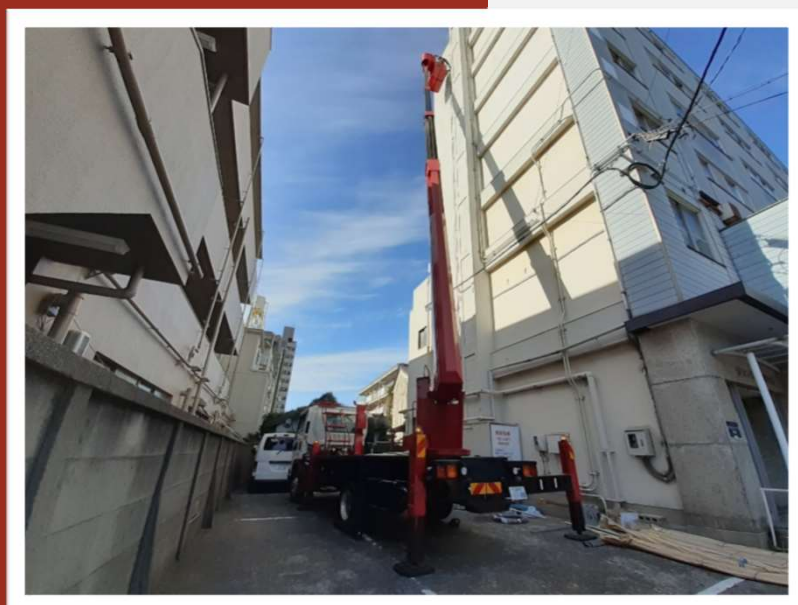
壁面配管敷設の状況
